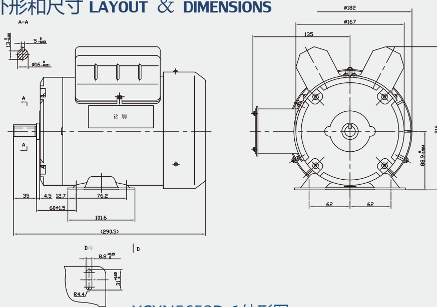
YCYN5652D-1外形图
