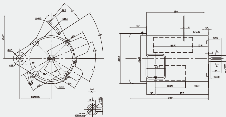
YCYGL8052外形图
