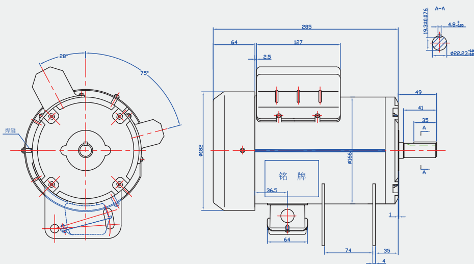
YCYN5692D-3外形图
